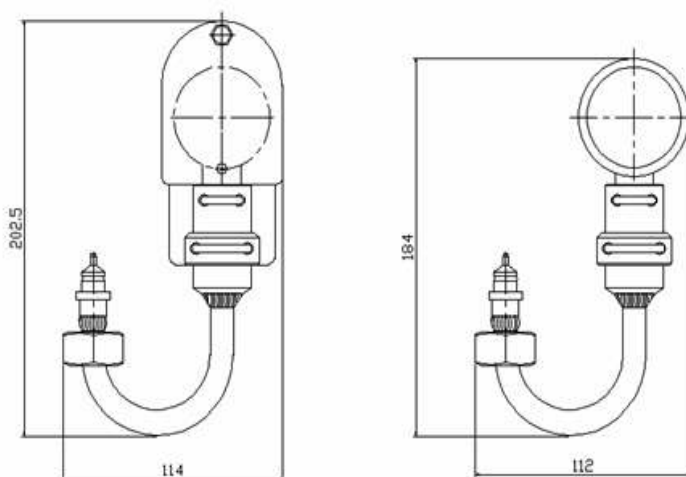
Výkr. PT001-22.2 (sříňka)
