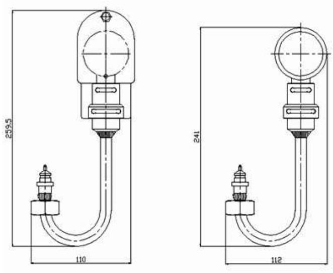
Výkr. PT001-21.2 (skříňka)
